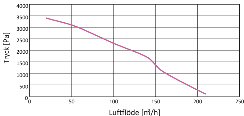
Fläktdiagram (totaltryck som funktion av volymflöde)
